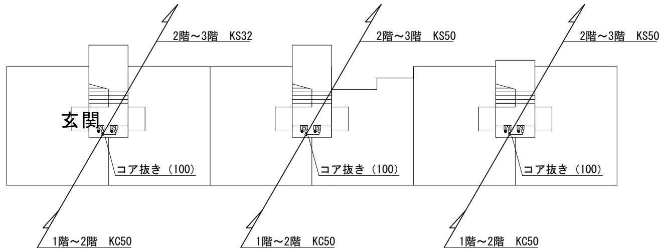
8号棟 2~3階平面図
