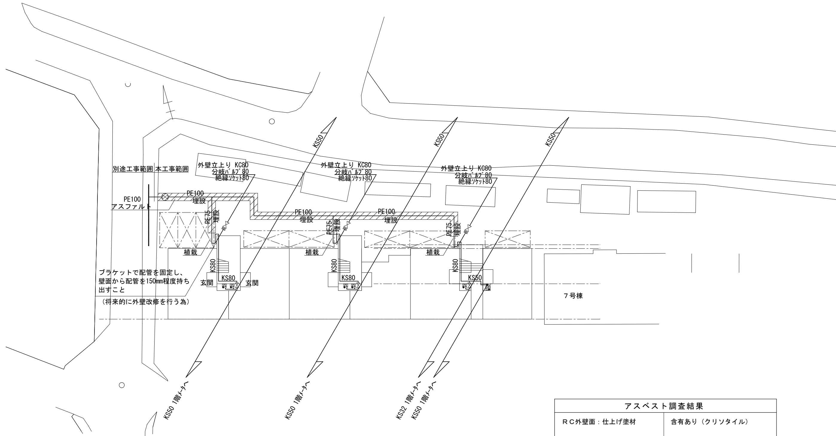
8号棟 1階平面図
