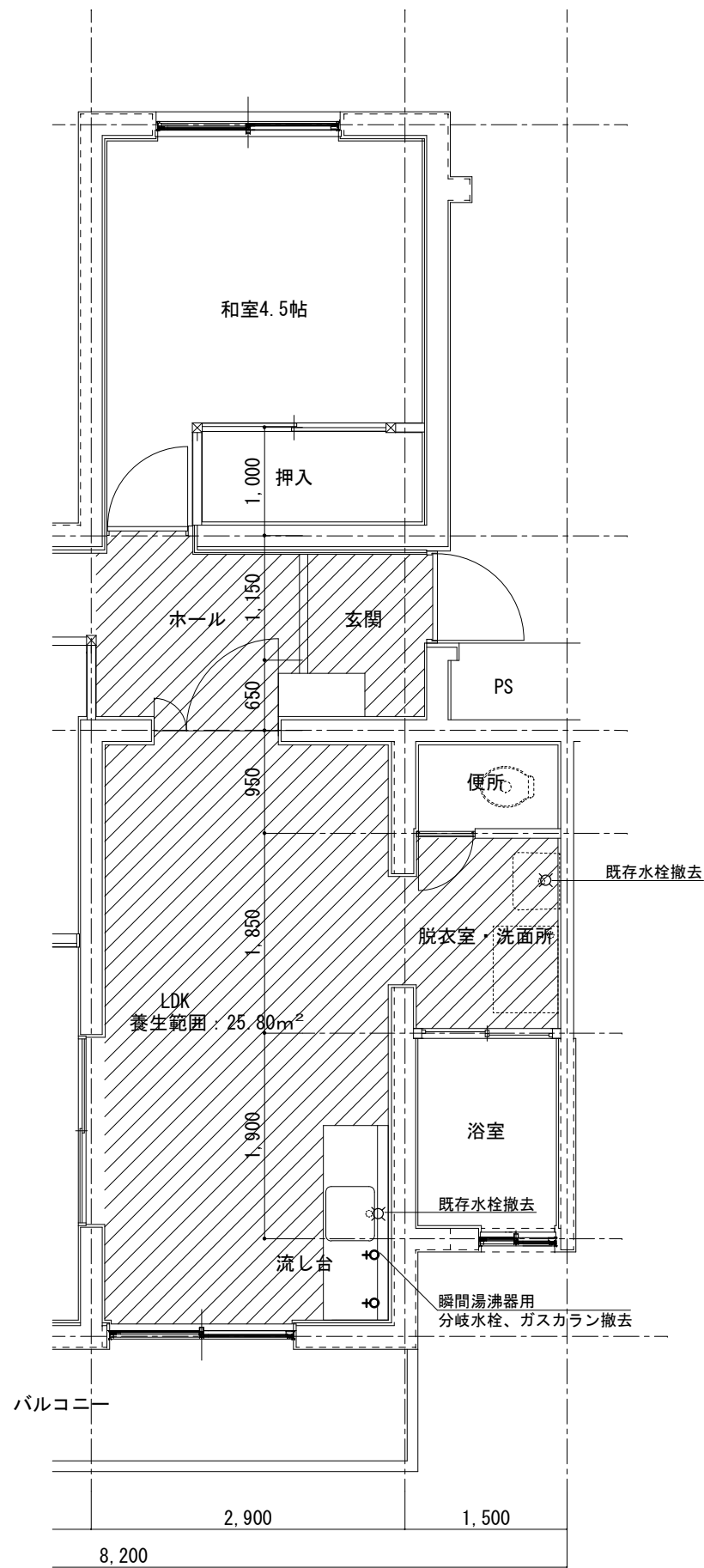
改修前機械設備図
