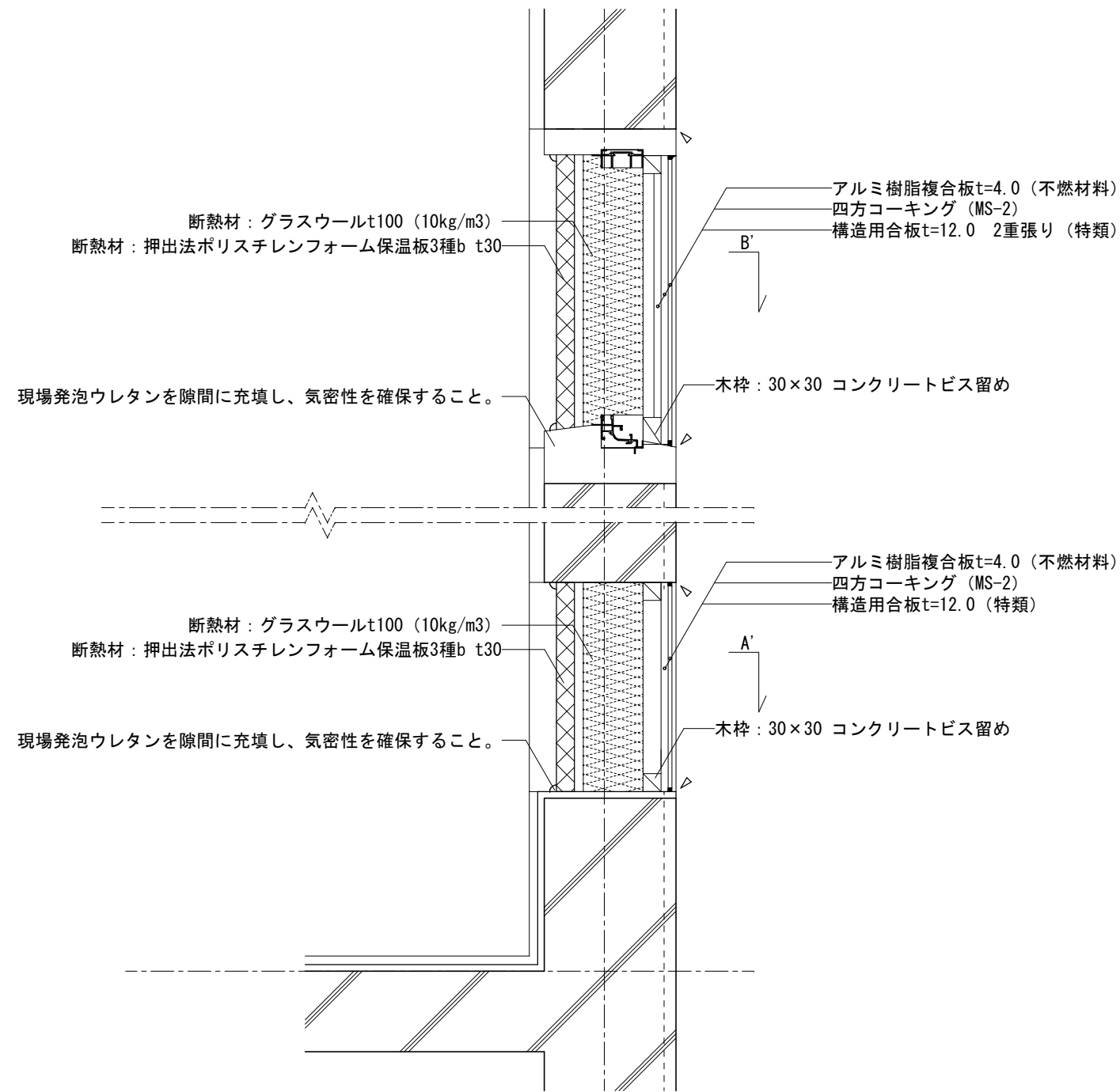
既存開口部 塞ぎ処理部詳細図 1/10
