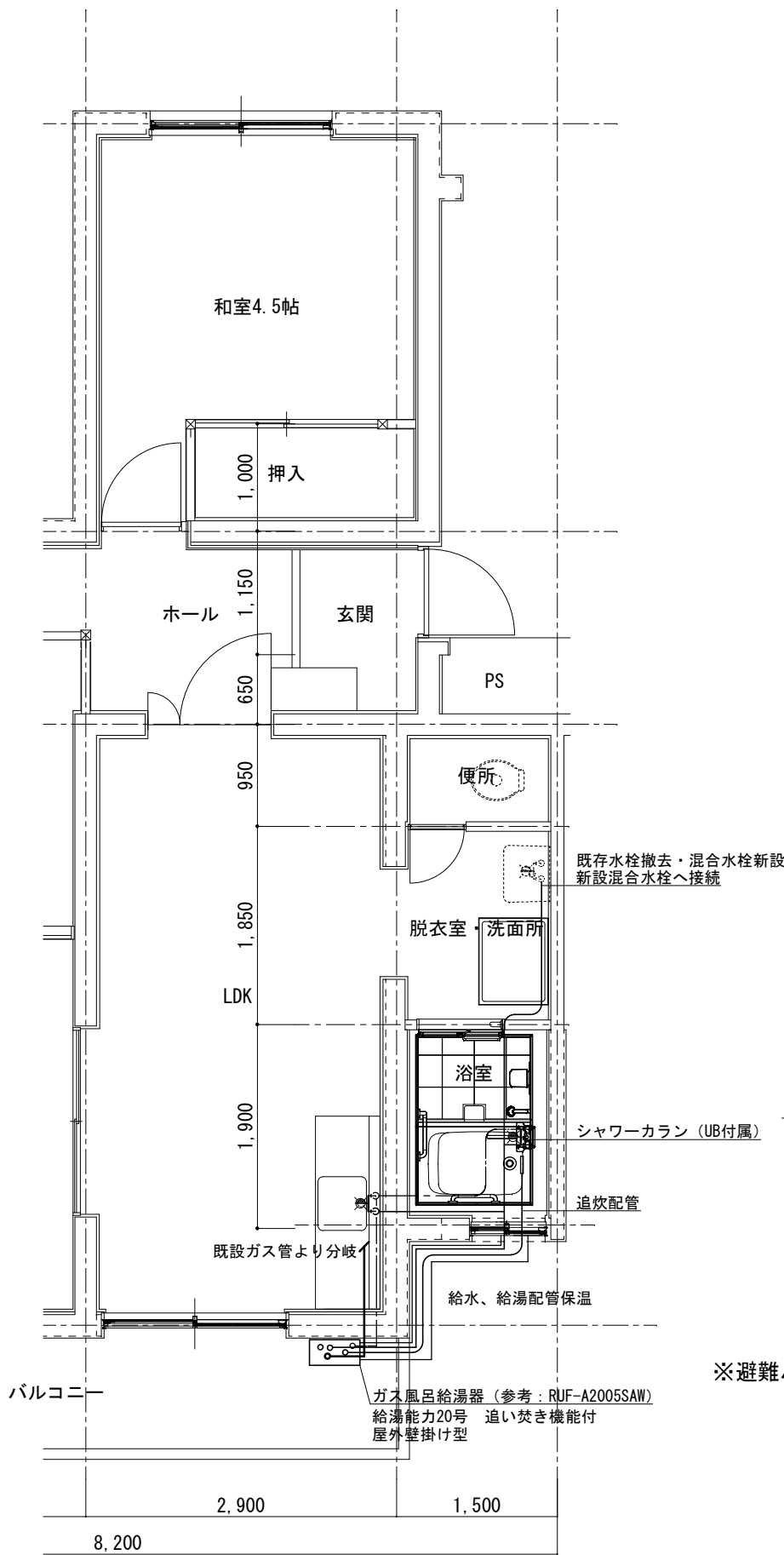
改修後機械設備図
