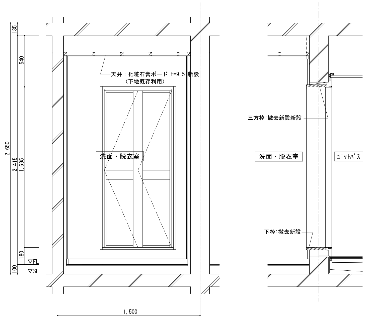
浴室出入口周り詳細図 1/20
